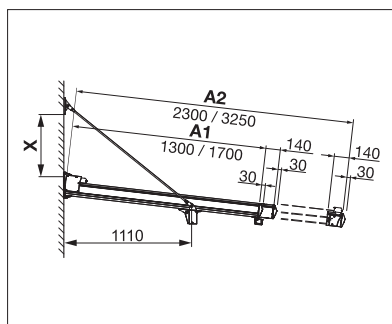
Montage mural avec barre de traction
