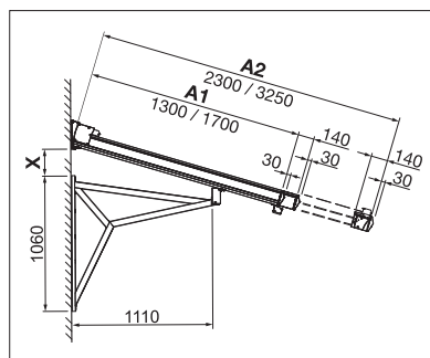
Montage mural avec console d'angle
