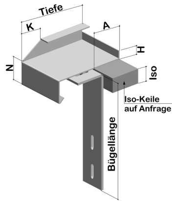
Pfeilerausschnitt mit Stehbord 2-seitig
