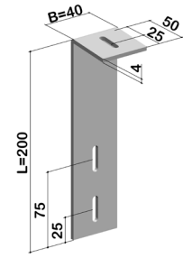
Langlöcher 6.5 x 26mm
