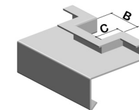
Pfeilerausschnitt mit Putzbord 3-seitig
