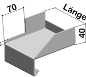
Stehbord St40-7/70
