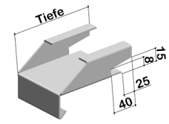
Spez. Klinkung Wetterschenkel KWS 40-25/8-15
