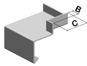
Pfeilerausschnitt mit Stehbord 2-seitig
