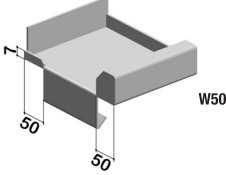
Wasserabweiser zu Steh- und Putzbord W7/50
