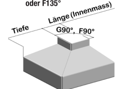
Gehrung mit Dilatation beliebige Winkel G90°, Formecke F90° oder F135°
