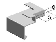
Pfeilerausschnitt mit Putzbord 2-seitig
