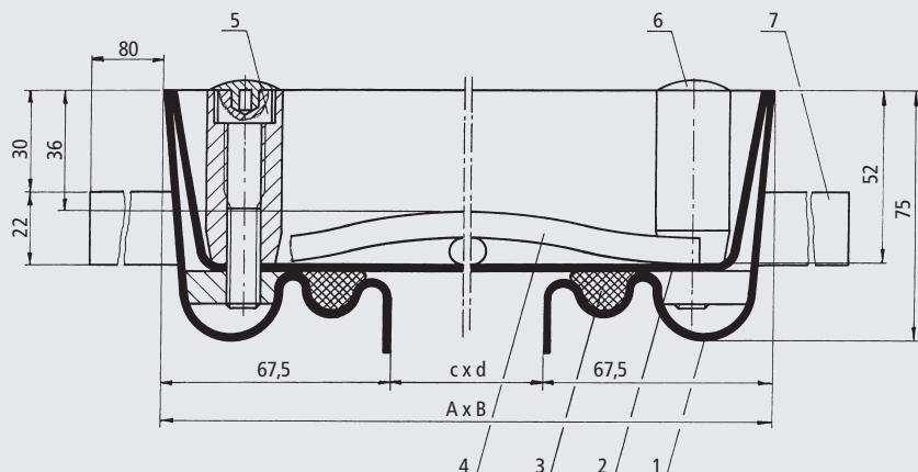
Type BVE acier spécial, Échelle 1 : 2,5
