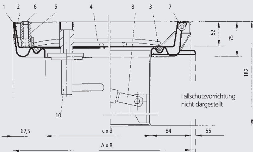
Typ BV-GDZ Stahl, Maßstab 1 : 5
