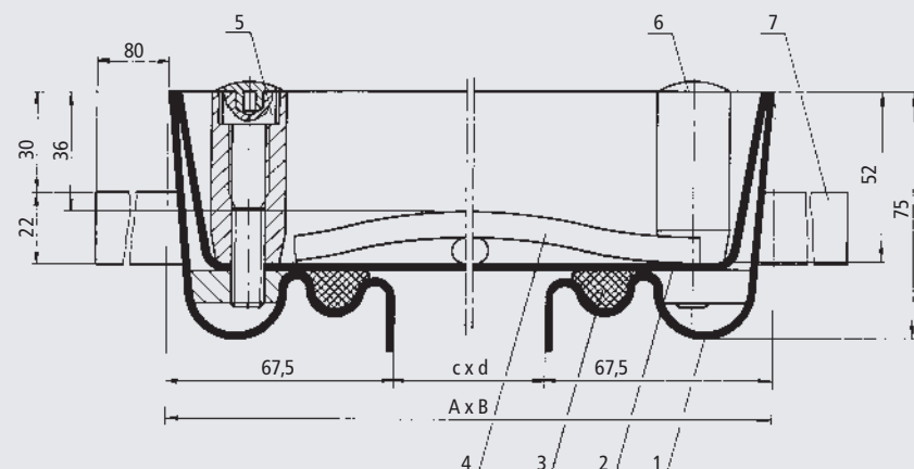
Typ BVE Edelstahl, Maßstab 1 : 2,5
